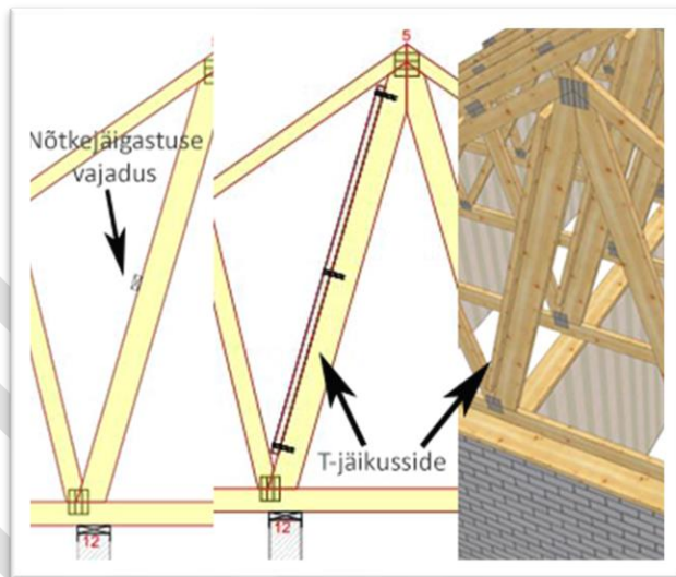
Joonis 16 T-nõtketugi
