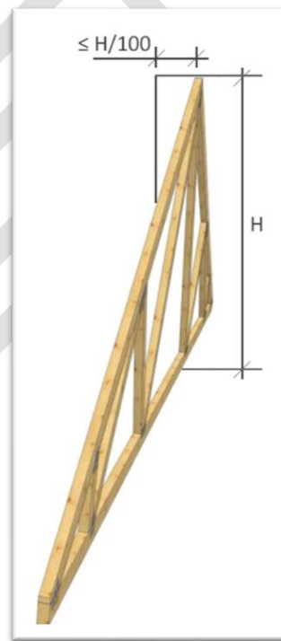
Joonis 11 Fermi maksimaalne lubatud kõrvalekalle
