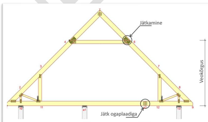
Joonis 8 Katusefermi veokõrgus ja vööde jätkamine
